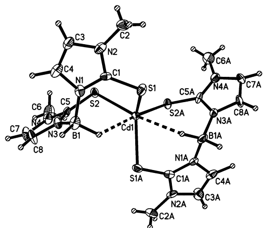
Figure 2. Molecular structure of \text{Cd}[\text{Bm}^{\text{Me}}]_2 . Selected bond lengths (Å) and angles (deg): \text{Cd1}-\text{S1} 2.5089(13), \text{Cd1}-\text{S2} 2.5716(11), \text{Cd1}-\text{H} 2.582, \text{S1}-\text{C1} 1.735(4), \text{S2}-\text{C5} 1.708(5); \text{S1}-\text{Cd}-\text{S1A} 114.55(6), \text{S1}-\text{Cd1}-\text{S2A} 104.31(4), \text{S1}-\text{Cd1}-\text{S2} 119.21(4), \text{S2}-\text{Cd1}-\text{S2A} 94.34(5).
